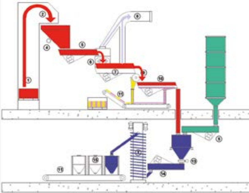
Séparer / Scalper / Cribler
