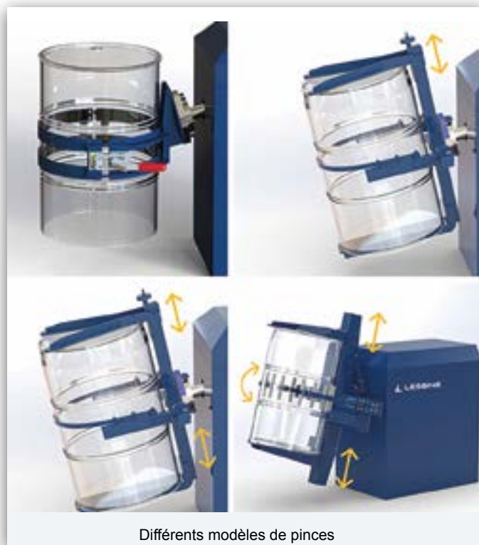
Pince manuelle ou à commande électrique 1 axe 2 formats (50 à 250l ou 100 à 250l)
