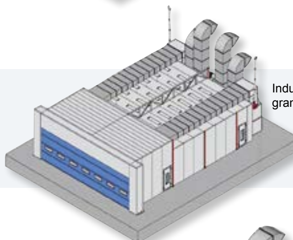
Industrie avec convoyage
