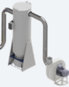
Unité de micronisation MIC6 30 à 90 kW
